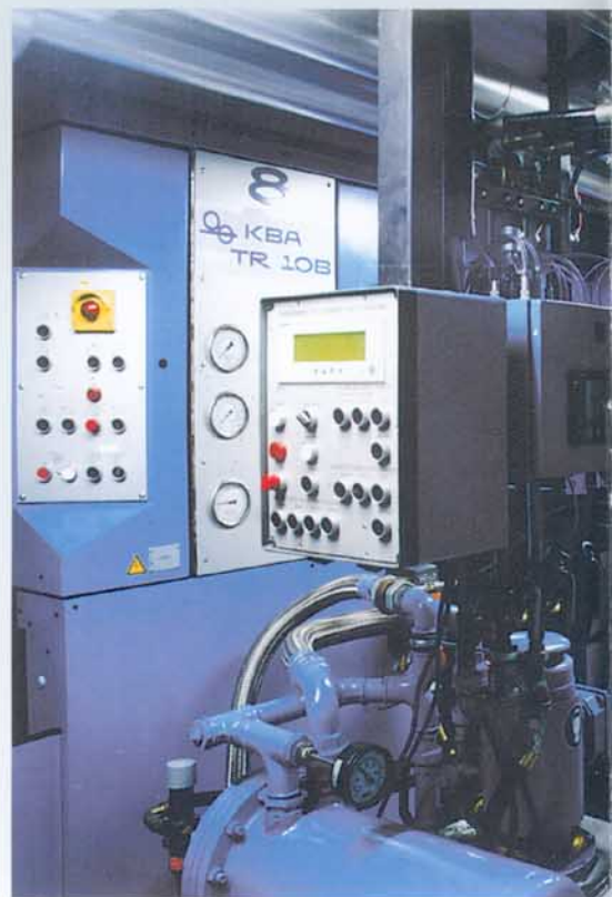
KBA TR10 Tiefdruckrotation ausgerüstet mit MITEX Presseur
