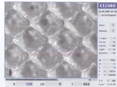
Lasergrafierte 70 Shore D Walzenoberfläche
